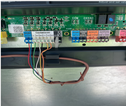
Unitwiring.jpeg
