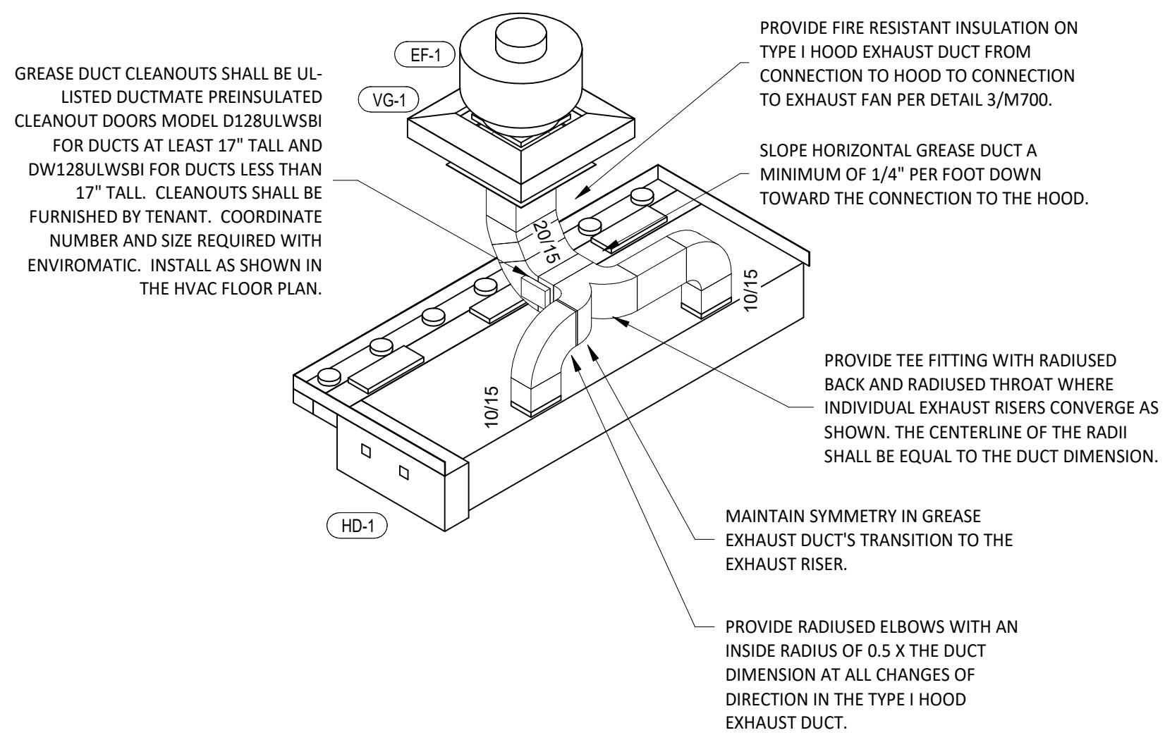
8 HOOD EXHAUST ISOMETRIC N.T.S.
