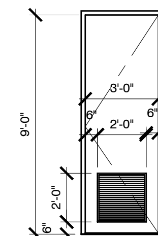
A BLDG STANDARD DOOR BLDG STANDARD FRAME
