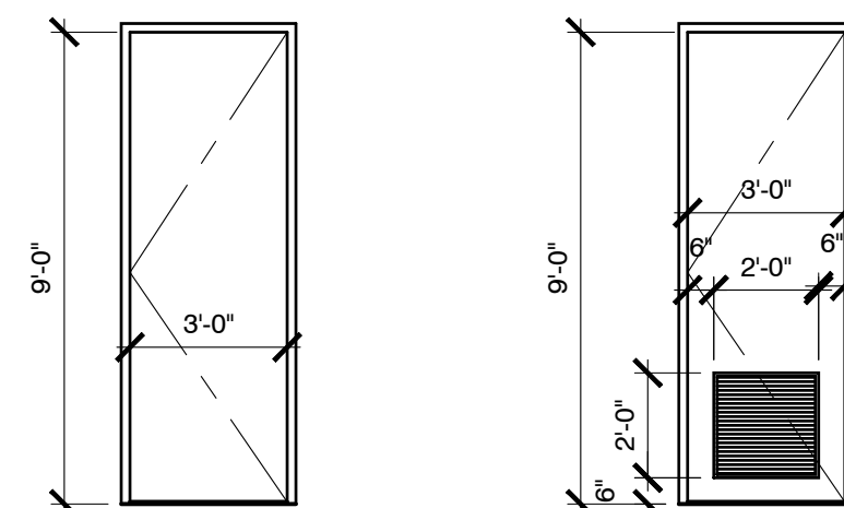
A BLDG STANDARD DOOR BLDG STANDARD FRAME
