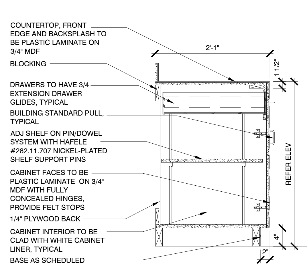
05 BASE CAB. SECTION SCALE: 1" = 1'-0"
