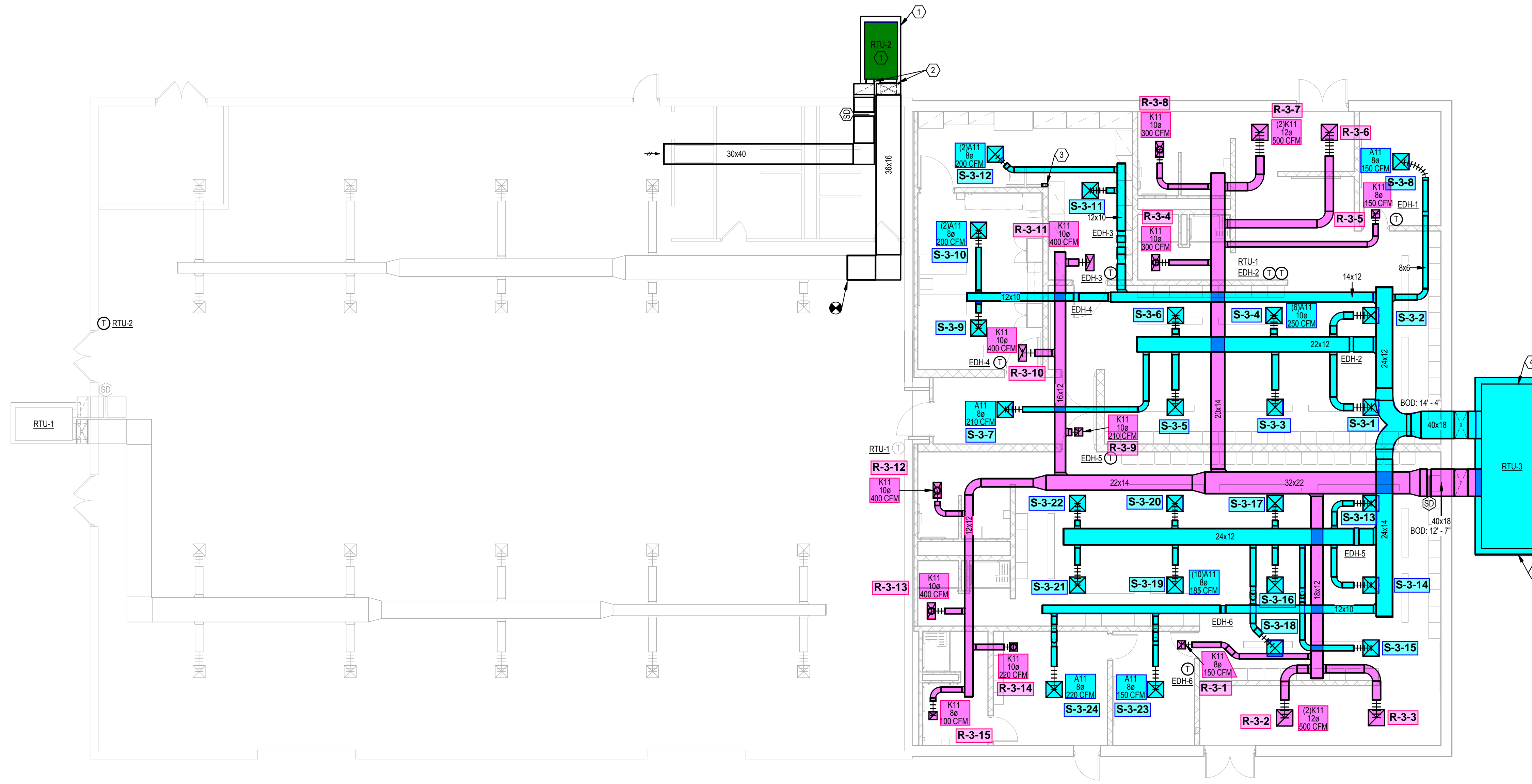
1 HVAC LEVEL 1 SCALE: 1/8" = 1'-0"
