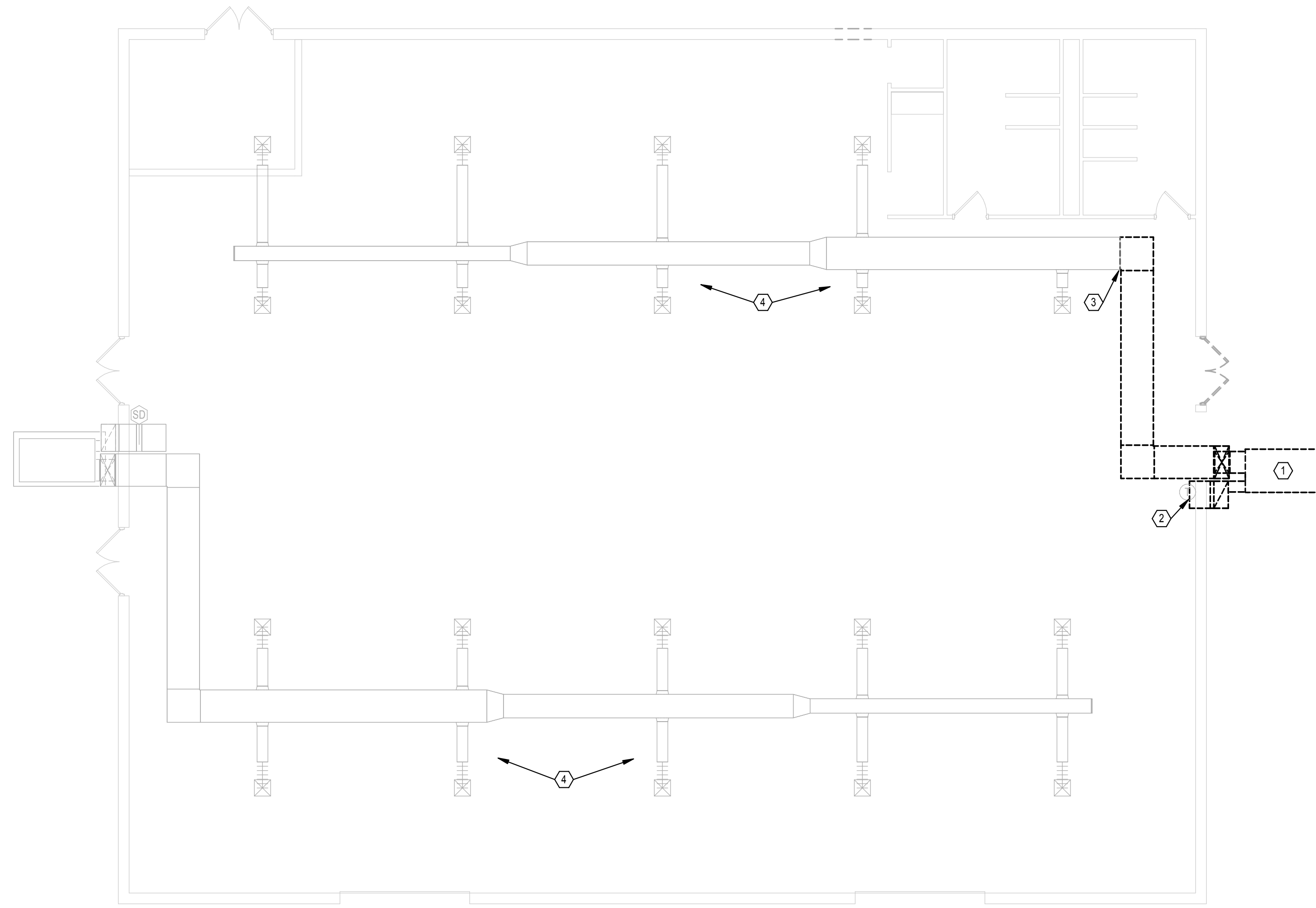
1 HVAC LEVEL 1 SCALE: 1/8" = 1'-0"
