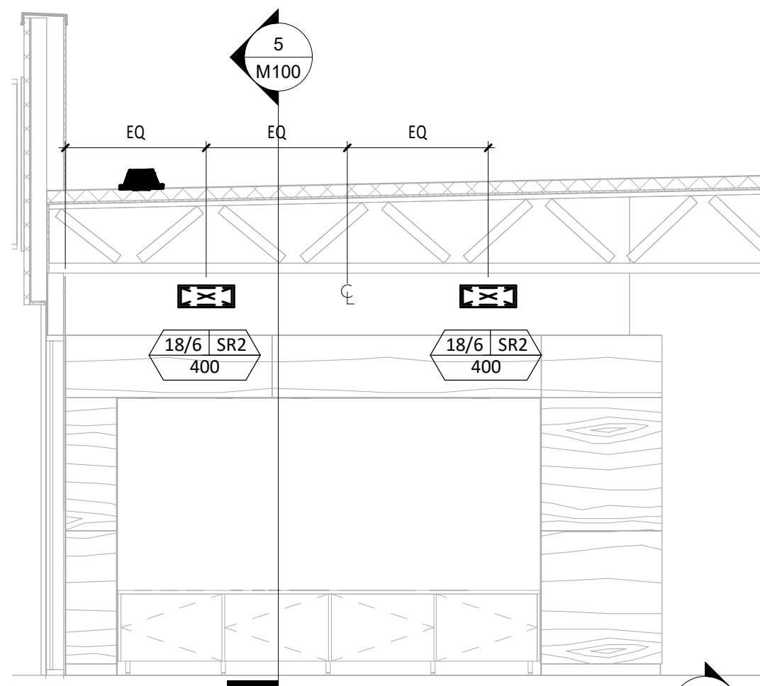
4 M100 1/4" = 1'-0"
