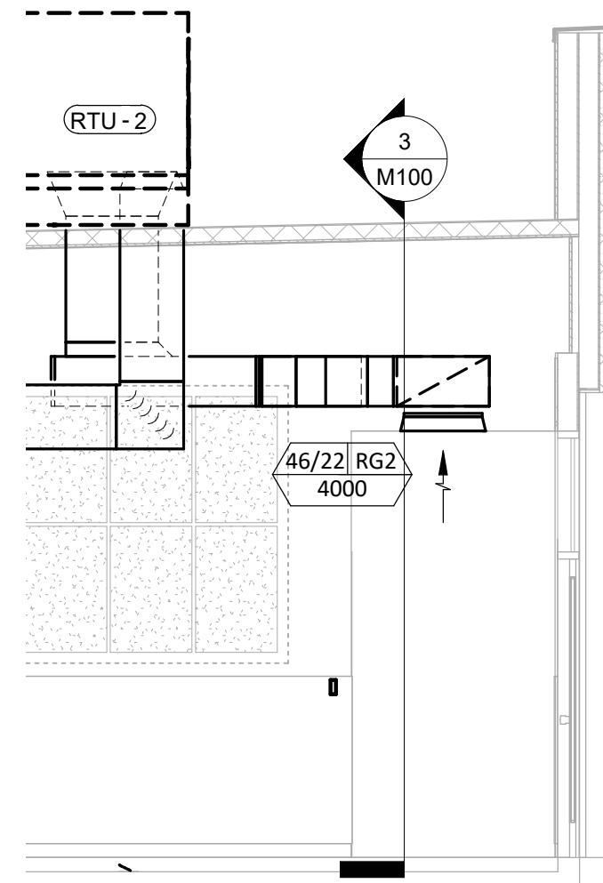
6 M100 1/4" = 1'-0"
