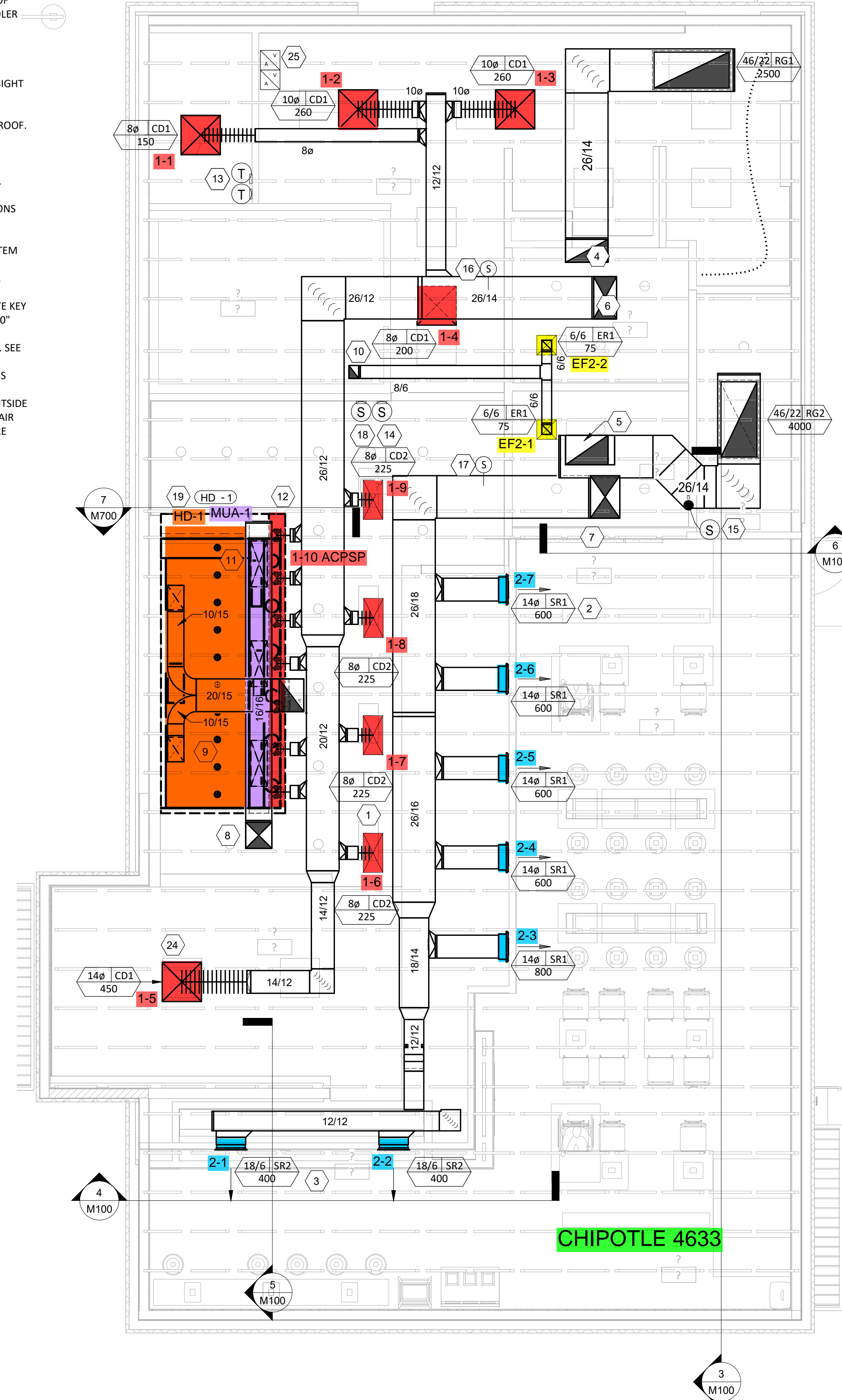
1 M100 1/4" = 1'-0"
