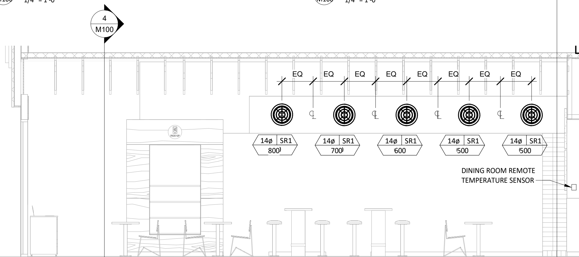
3 M100 1/4" = 1'-0"
