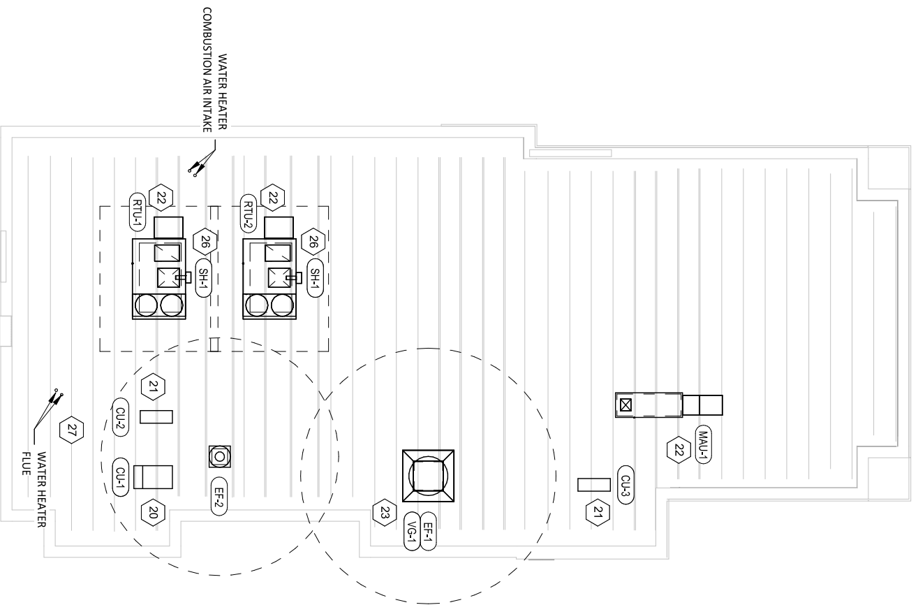
2 M100 1/8" = 1'-0"
