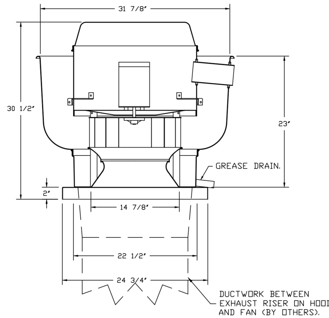
FANS #1 (EF-1), #2 (EF-2) - DU85HFA EXHAUST FAN
