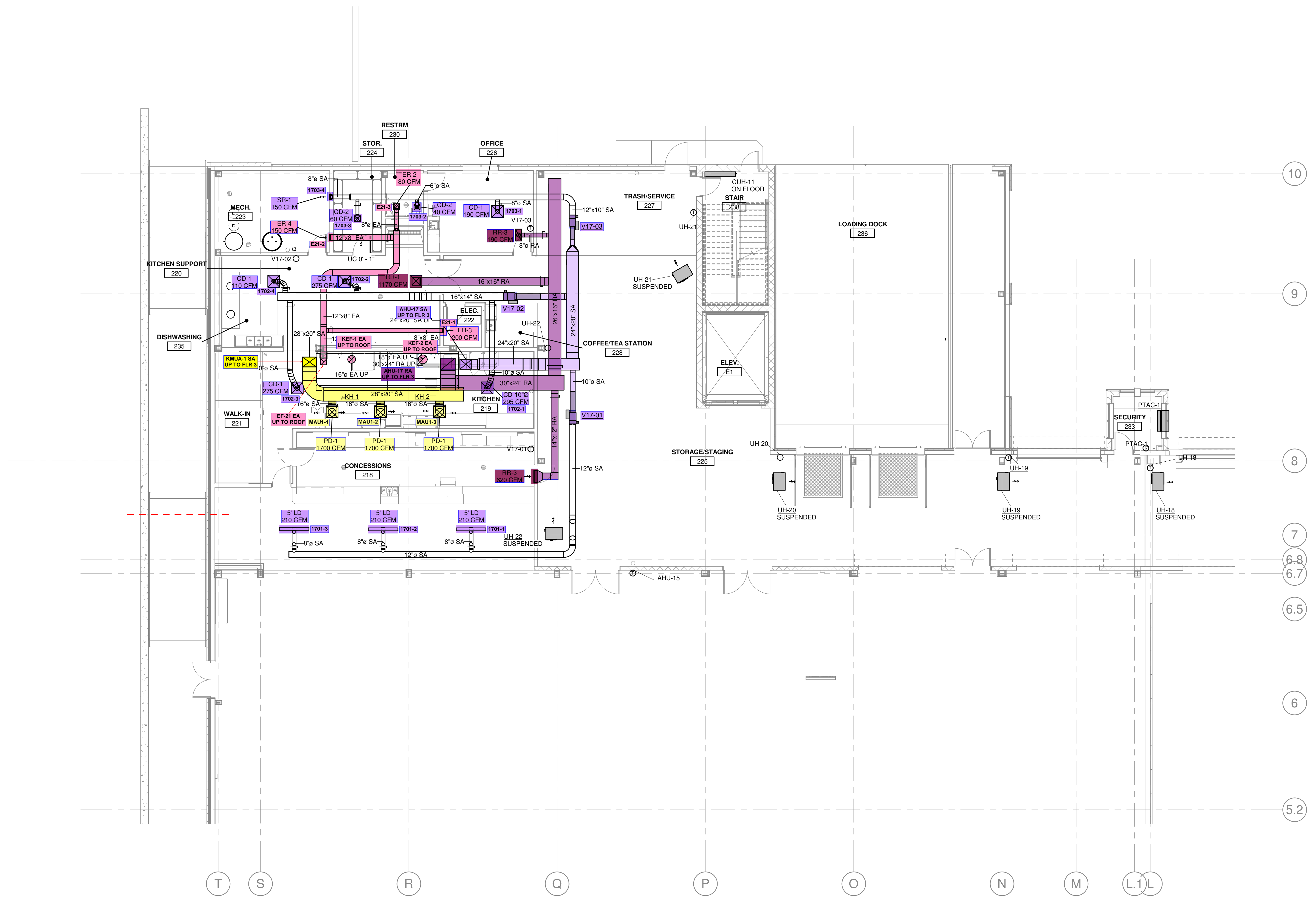
1 M-1.34B 1/8" = 1'-0"
