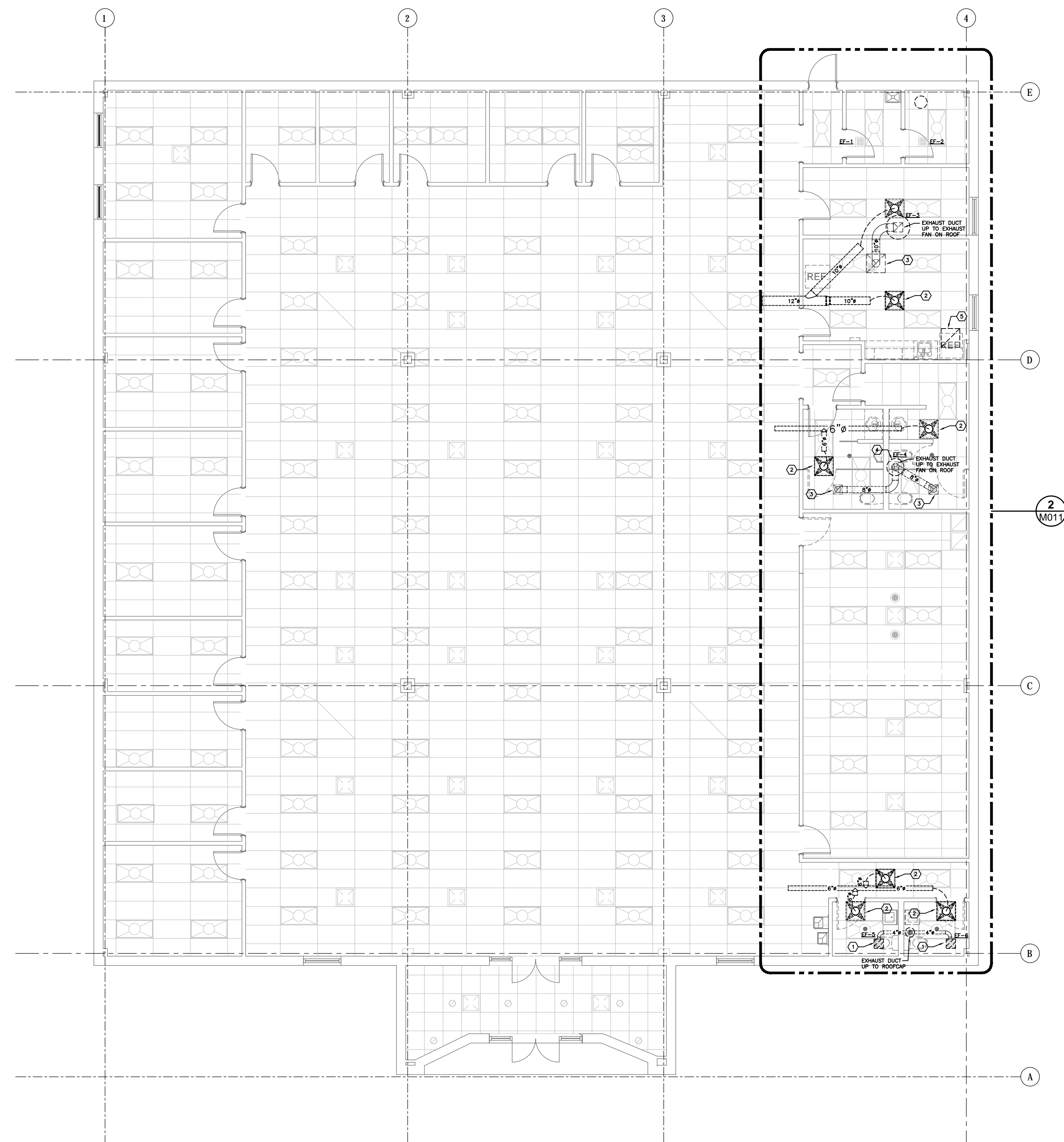
1 HVAC DEMOLITION PLAN M011 SCALE: 1/8" = 1'-0"
