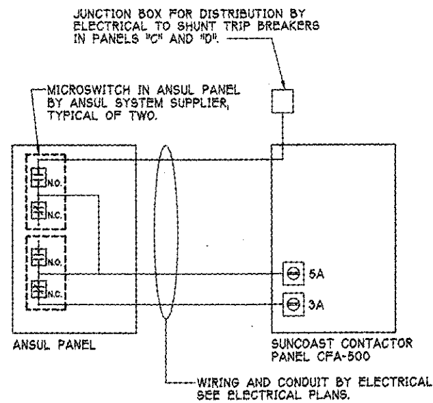
2 ANSUL WIRING DIAGRAM M3 SCALE: NONE
