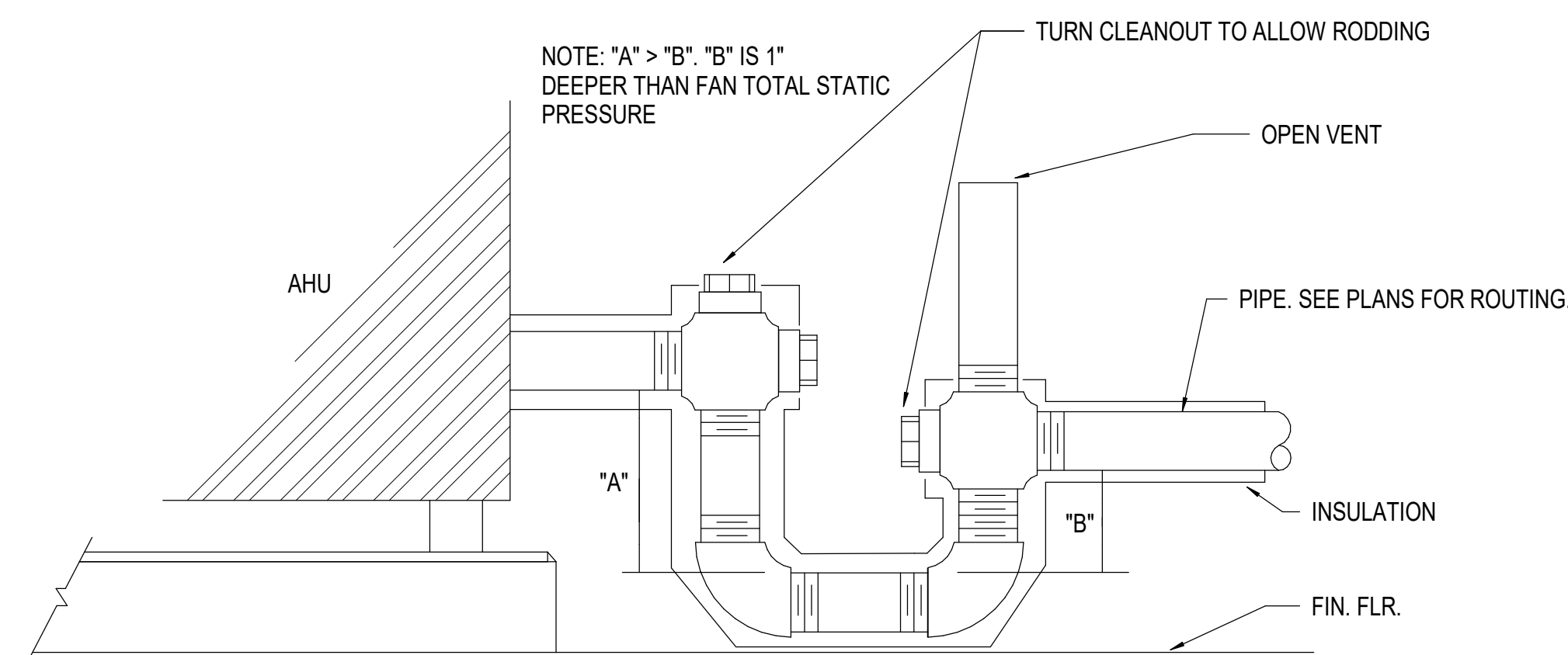
A3 BLOW-THRU AHU CONDENSATE DRAIN DETAIL N.T.S.
