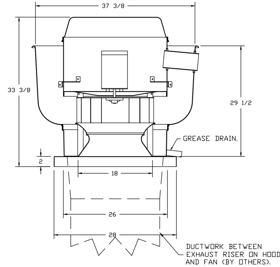
FAN #1 DU200HFA - EXHAUST FAN (EF-1)
