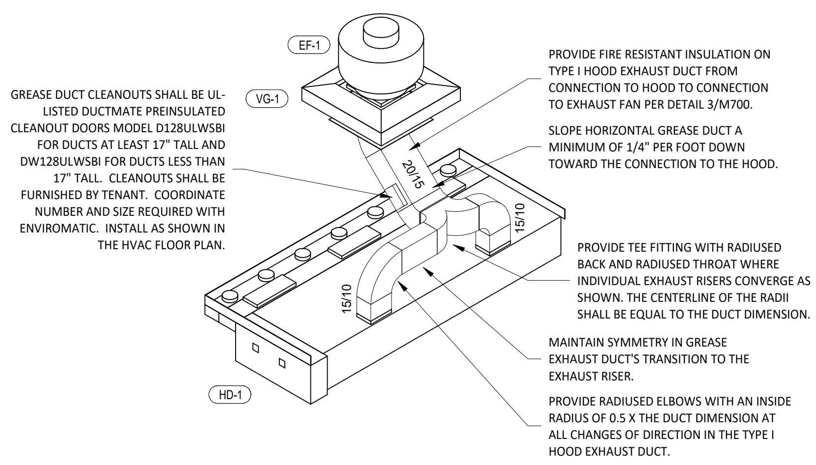
8 HOOD EXHAUST ISOMETRIC N.T.S.
