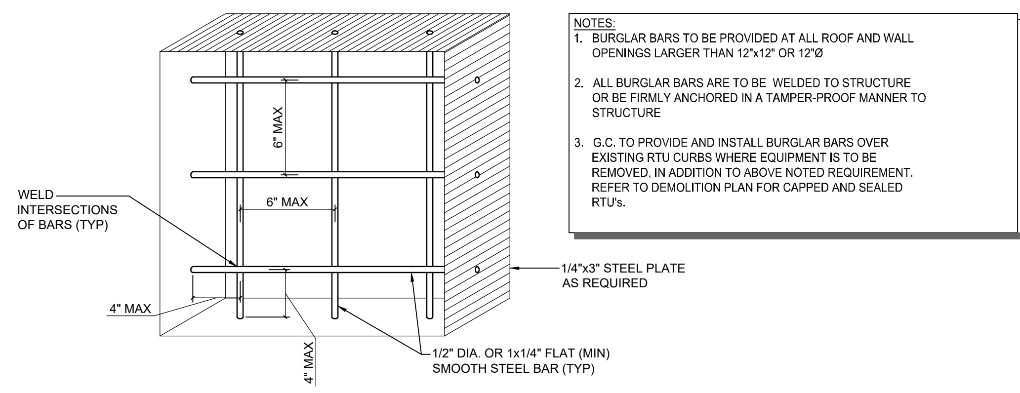
13 BURGLAR BAR DETAILS SCALE: NONE
