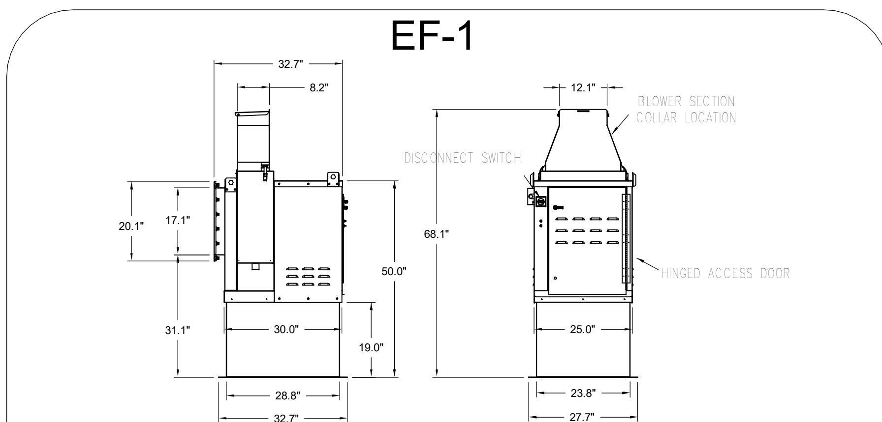
Halton KEFB Exhaust Fan
